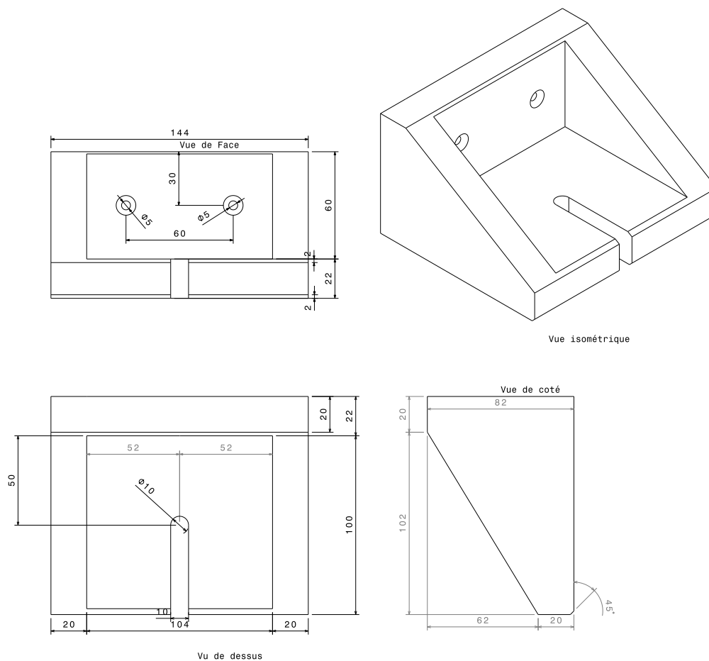
FIGURE 20 : Support de balise fixe (Modèle B)
