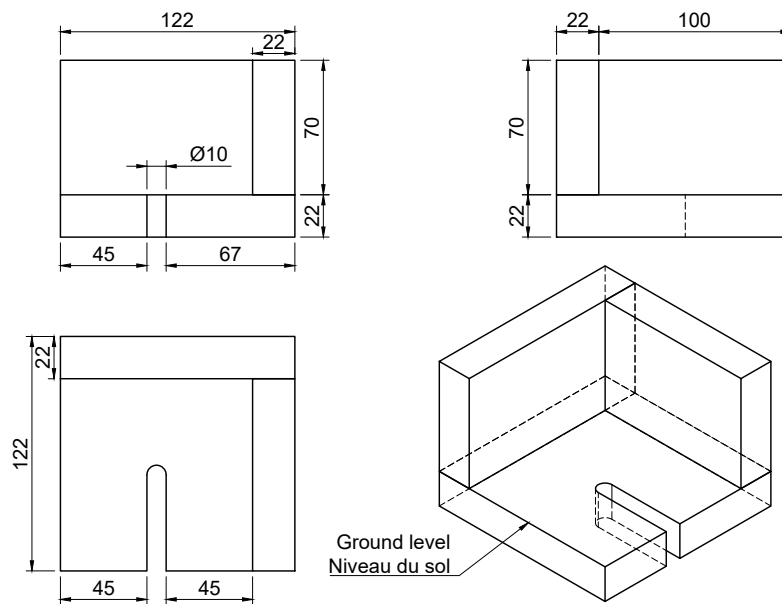
FIGURE 19 : Support de balise fixe droit (Modèle A)
